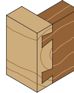
variabele-afstand zwaluwstaart
