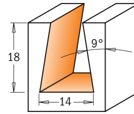
Schaal 1:1
